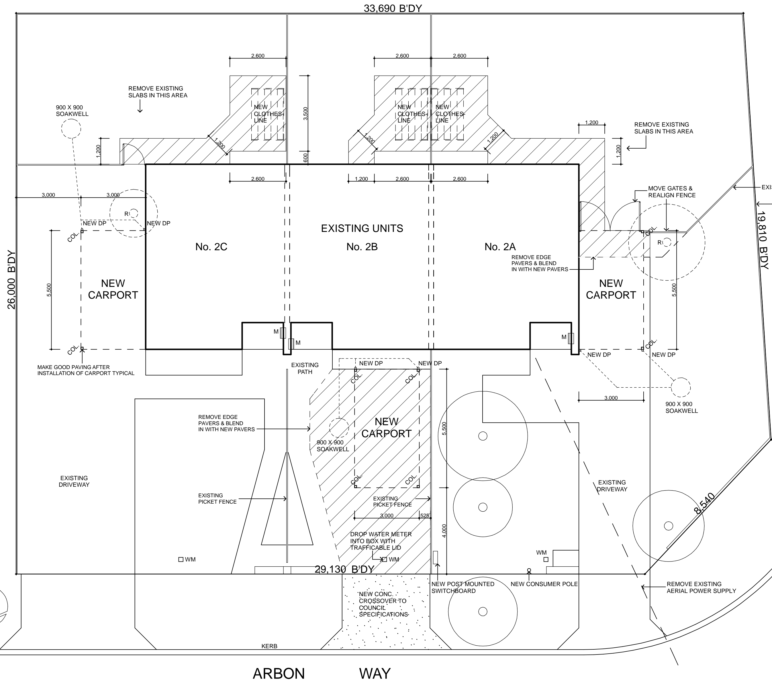
SITE PLAN 1 : 100
