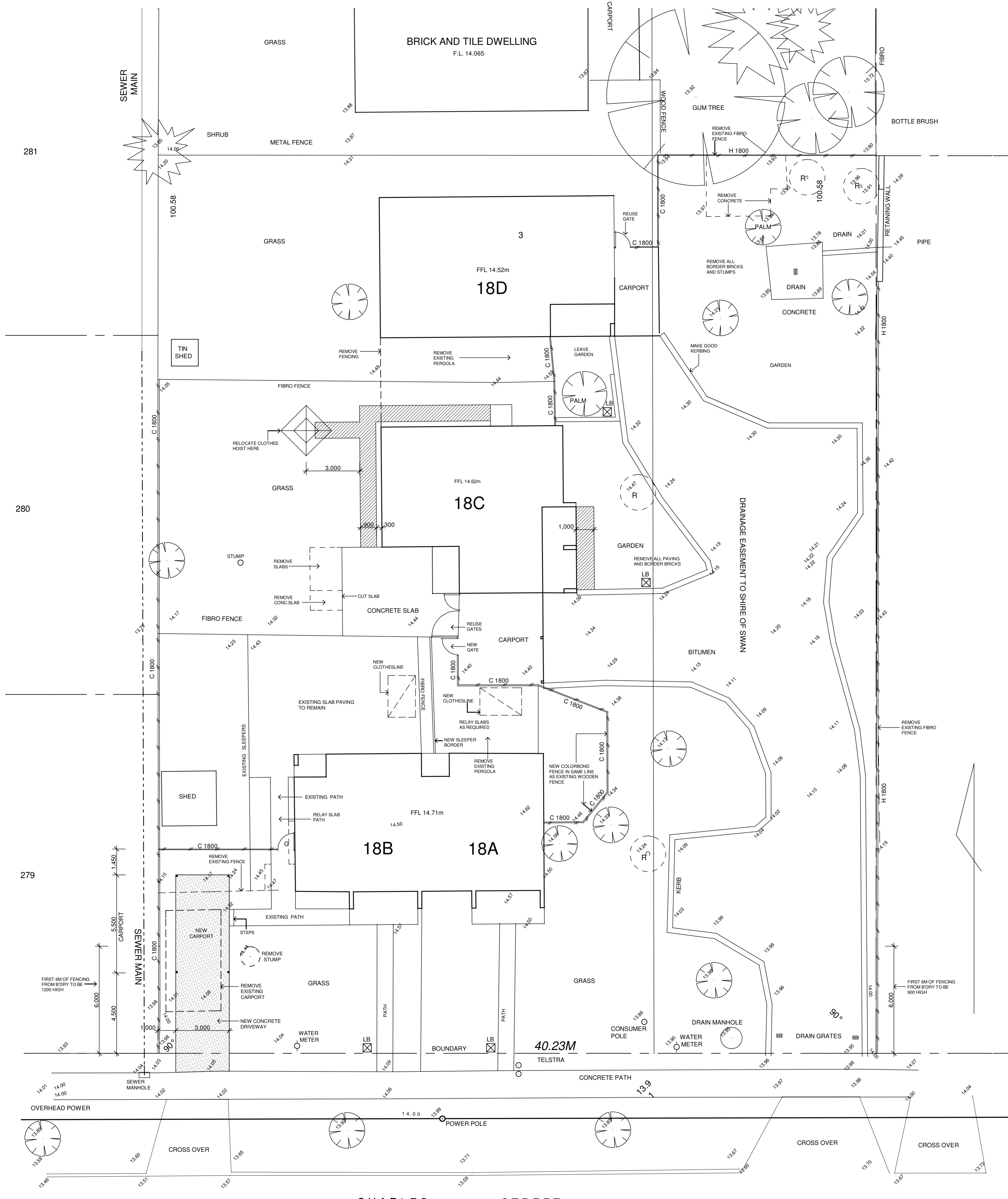
SITE PLAN 1:100
